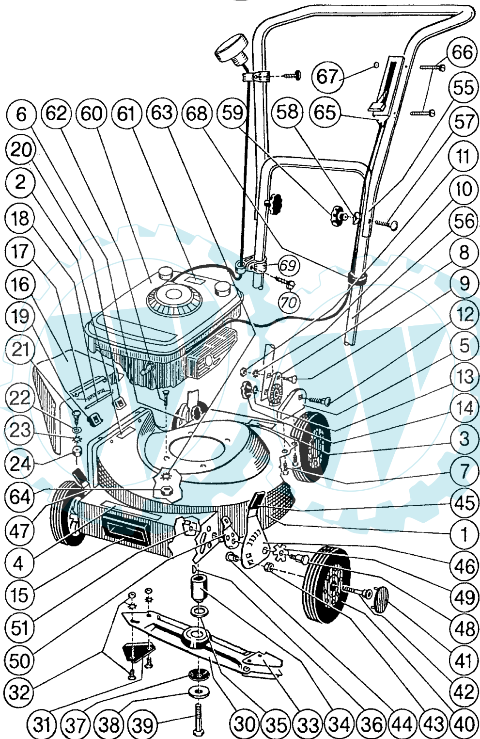
Roto - FOX 46 Typ 71132
